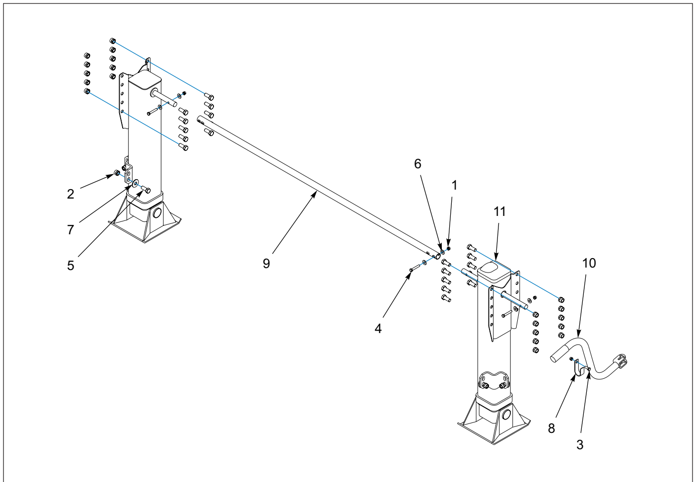
Figure 1-84: Jost 410
