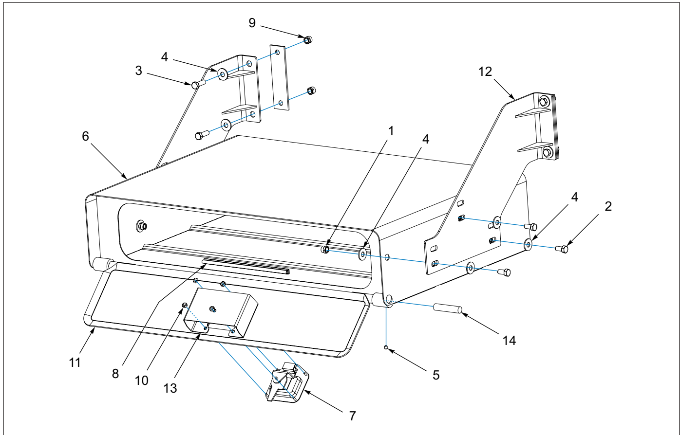
Figure 1-144: Toolbox Assembly-Steel/Aluminum Door
